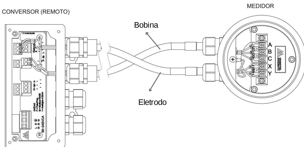
Figura 31 - esquema de ligação do transmissor 584TM ao conversor remoto 584TM
