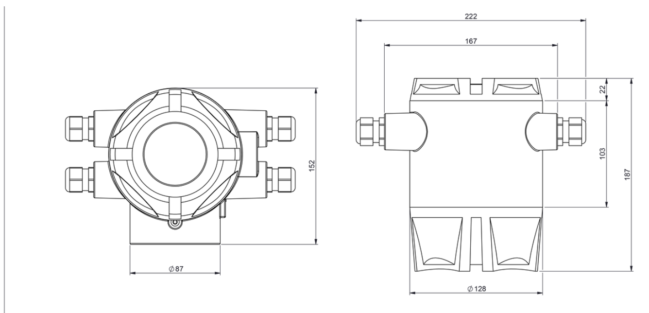
Figura 27 - Tipo compacto
